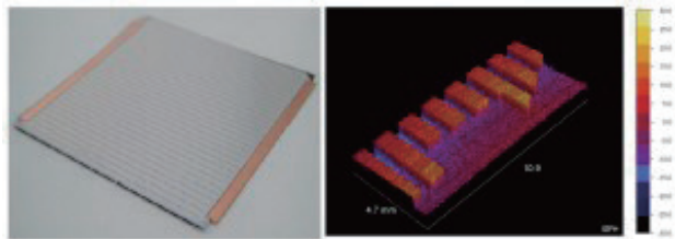
体硅太阳能硅片的结构化
